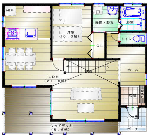
平面詳細図 1階
