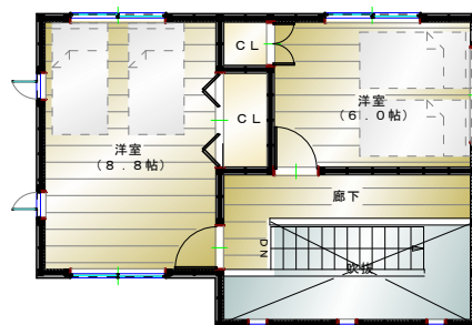
平面詳細図 2階
