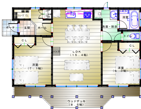
平面詳細図 1階
