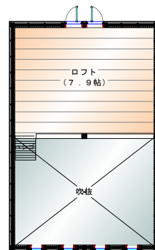
平面詳細図 2階
