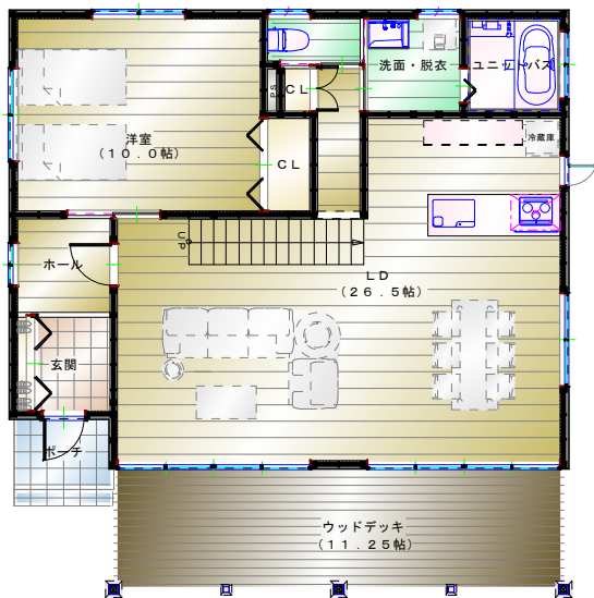
平面詳細図 1階
